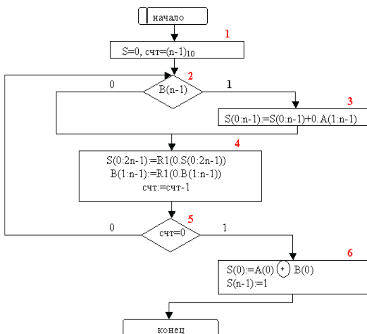
Рис. 1. Функциональная микропрограмма
