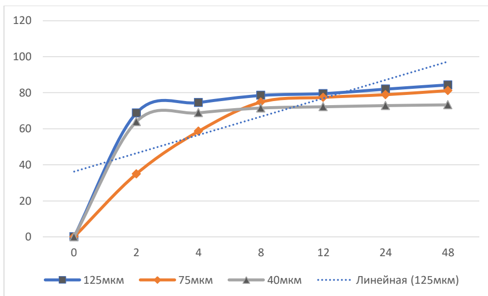
Рис. 1. Кинетика выщелачивания золота при различной тонине помола
