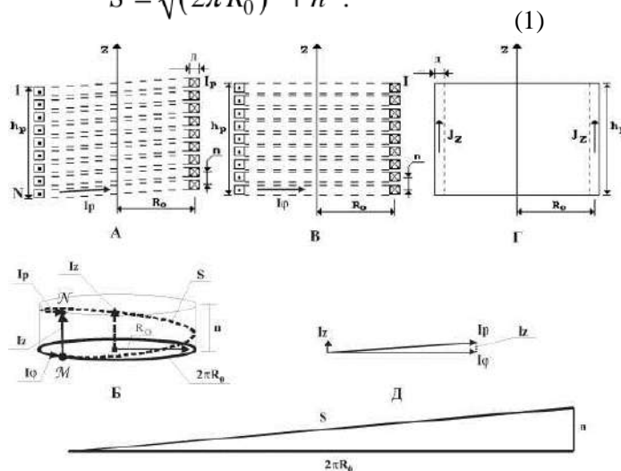
Рис. 1. Параметры токоограничивающего реактора
