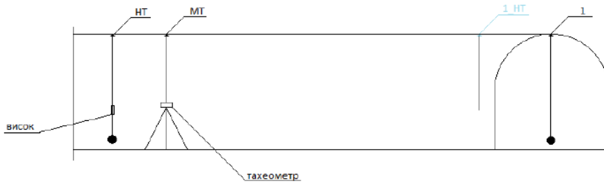
Рис. 2. Новая маркшейдерская точка для задания направления
