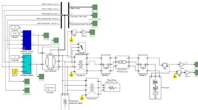
Рис.2. Модель малой ГЭС в Matlab/Simulink Параметры элементов электрической системы приведены в табл. 1.
