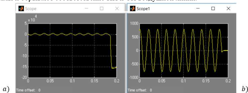
Рис. 6. Осциллограммы зависимостей: а) – разности потенциалов между СП и ИП; б) - ток в силовом проводе ПНТ в момент 0,182 с, когда произошёл обрыв провода
