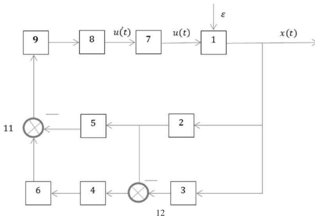
Рис.2. Упрощенная блок-схема
